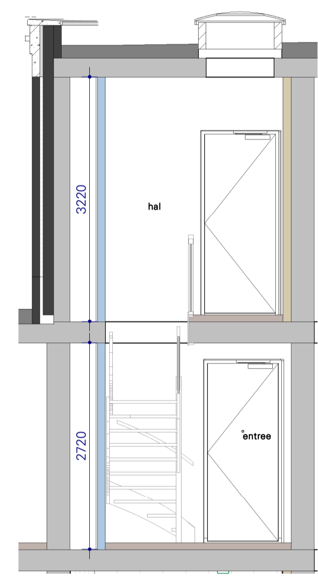
VK Doorsnede B - Blok E - bnr094
